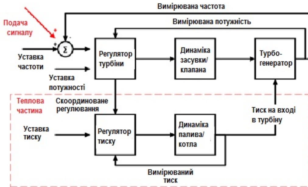
Рисунок 1. Приклад подачі сигналу регулятора
